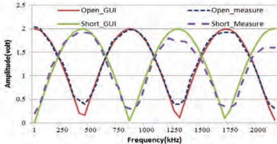
ภาพที่ 7 คลื่นยืนบนสายส่งขณะเปิดและลัดวงจร
